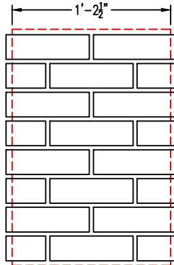
ELEVATION
